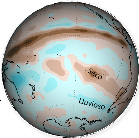
Precipitación
