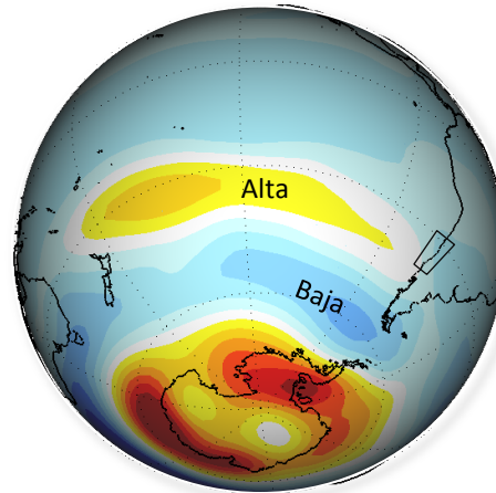
Presión (Z500)
