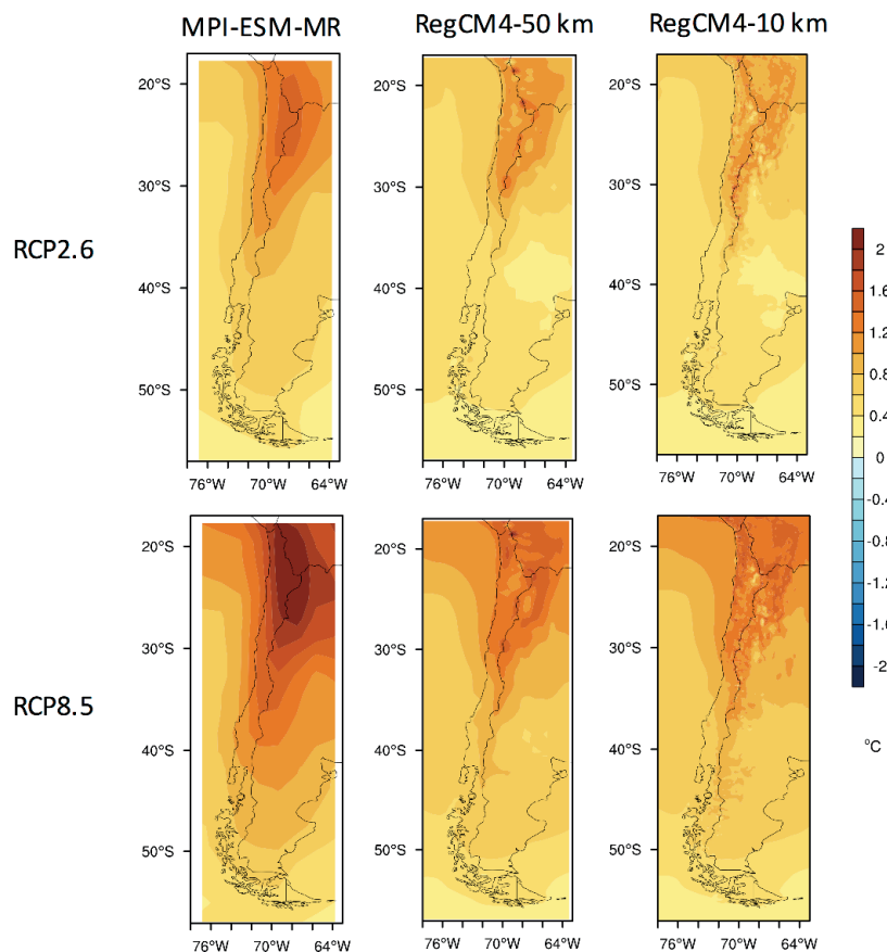
Figura 8: Mapas de cambio de temperatura (°C, anual) para el periodo 2021-2050, con respecto al periodo 1976-2005 basado en el modelo MPI-ESM-MR según los escenarios RCP2.6 (paneles superiores) y RCP8.5 (paneles inferiores).
